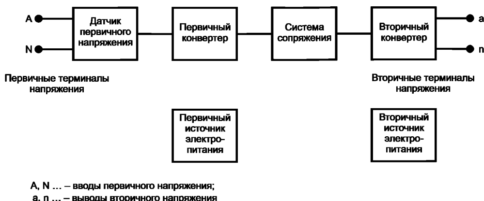
Рисунок 1 — Блок-схема заземляемого однофазного ЭТН
